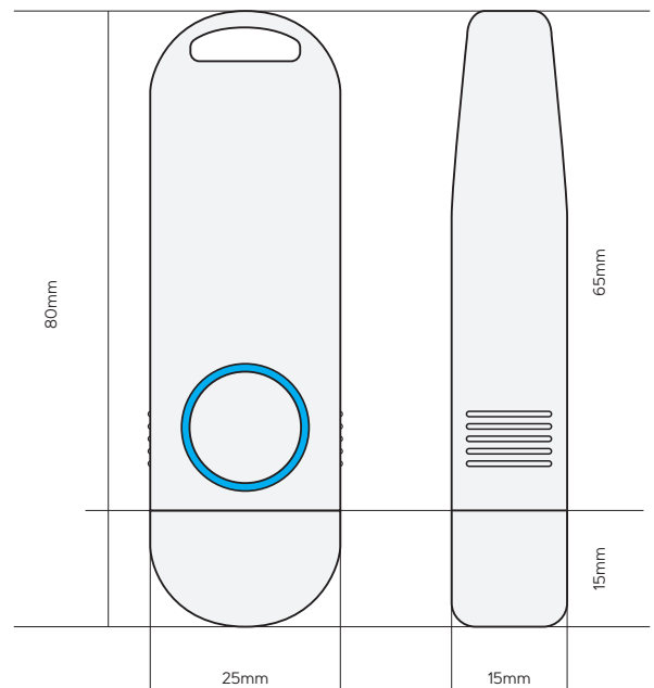
Beispiel eines individuellen ONEKEYs mit Ein-Knopf-Bedienung
